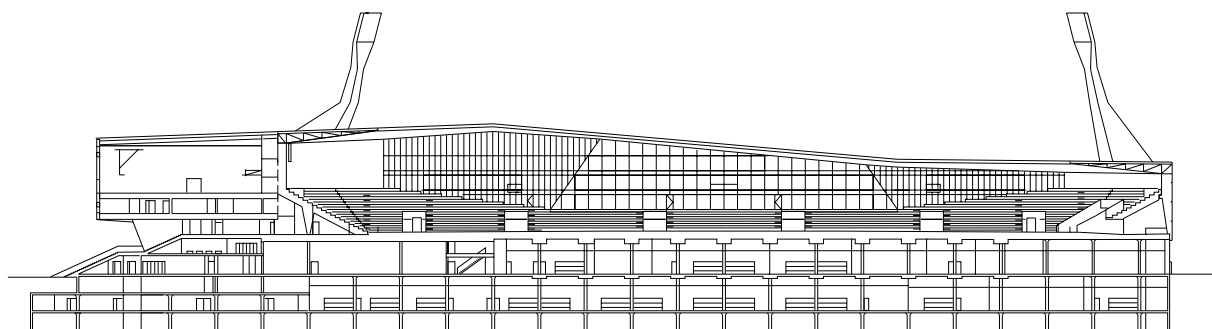
coupe longitudinale
