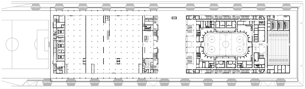
étage 0
